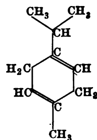
\gamma -Terpinene.
